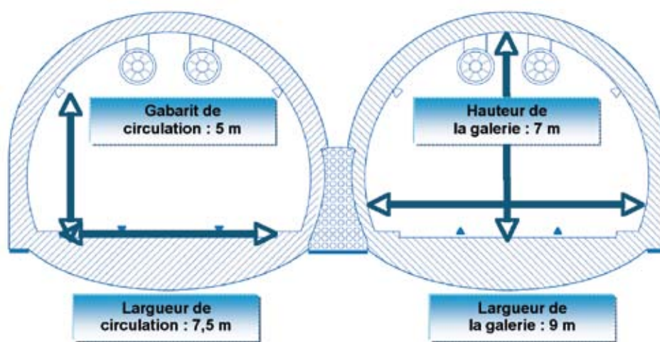
Coupe type du tunnel en rocher
